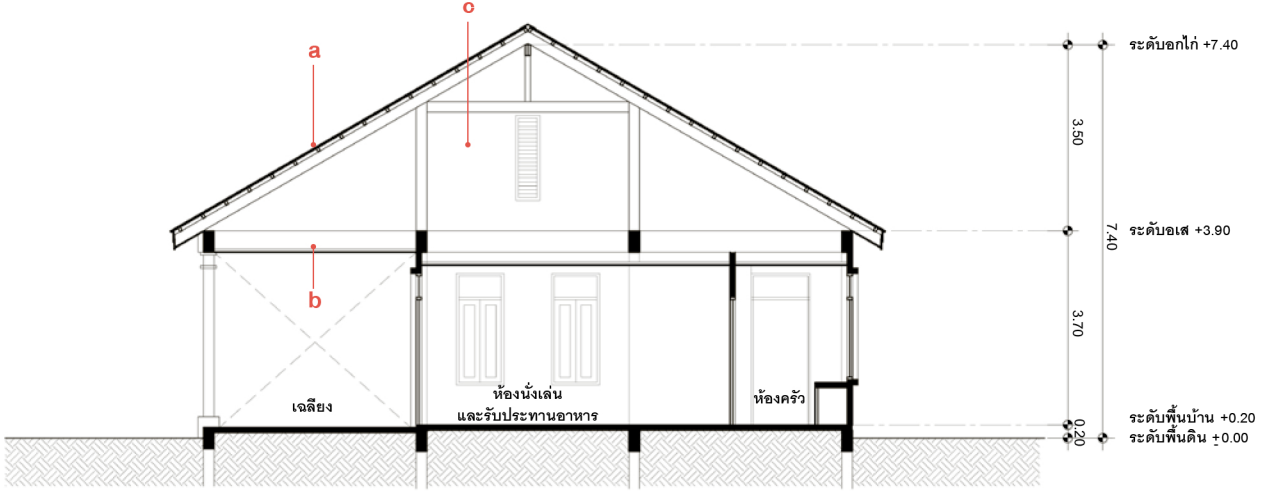
รูปตัด
